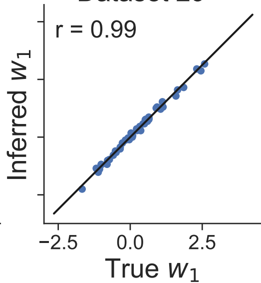
Dataset 29
