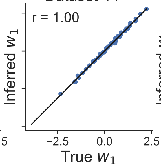
Dataset 44
